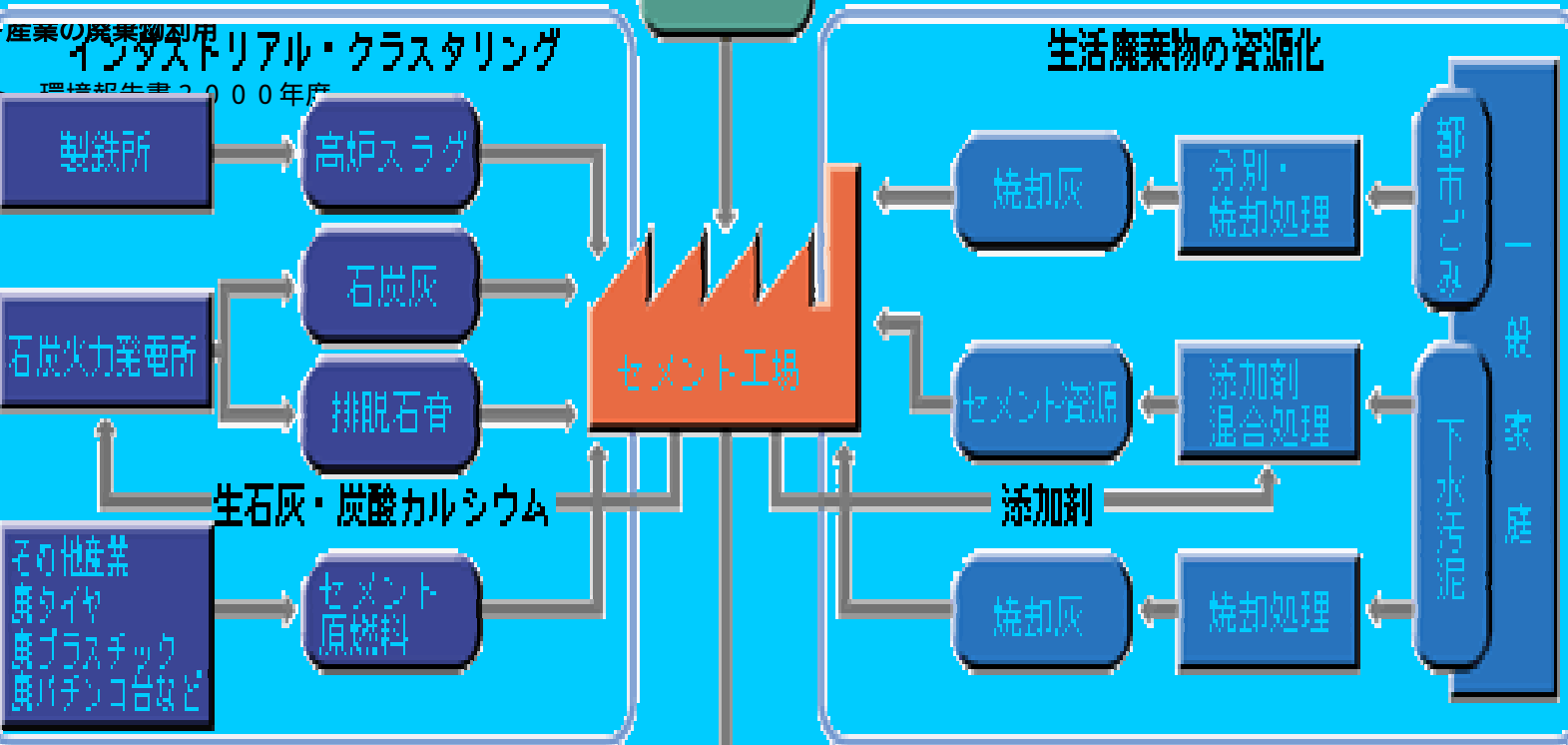
図2-1 セメント工場を中心とした資源循環型システム 太平洋セメント 環境報告書2000年度
